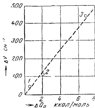
Рис. XVIII, 12. Зависимость между смещением частоты валентных колебаний \Delta\nu свободных гидроксильных групп поверхности кремнезема и разностью теплот адсорбции \Delta\bar{Q}_a на гидроксильированной и дегидроксильированной поверхности:
