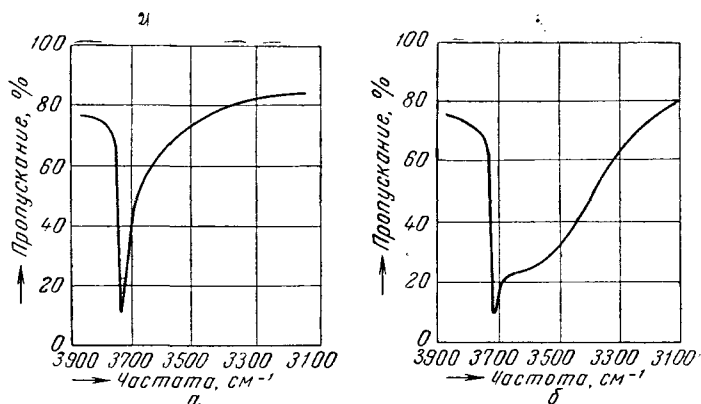
Рис. XVIII, 10. Инфракрасный спектр кремнезема: а—содержащего только свободные гидроксильные группы ОН; б—содержащего свободные и взаимосвязанные водородными связями гидроксильные группы.
