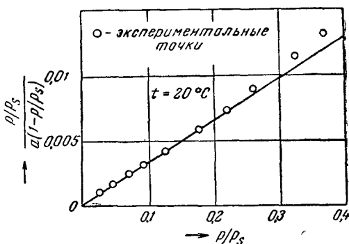
Рис. XVI, 9. Изотерма адсорбции пара бензола на поверхности графитированной сажи в координатах линейной формы уравнения БЭТ.
