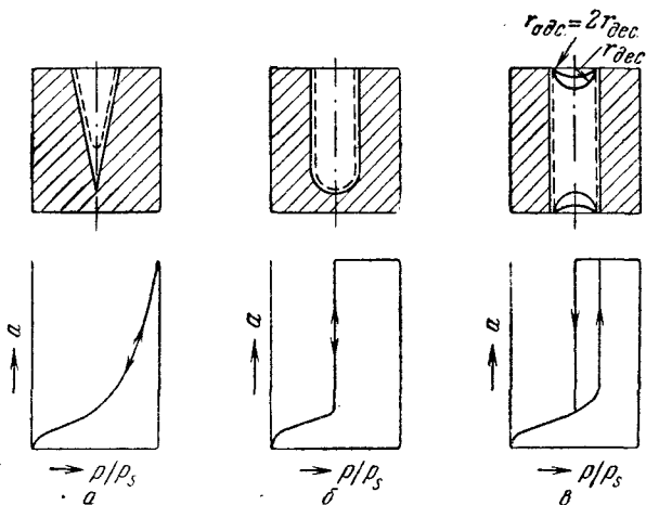
Рис. XIX, 5. Схема капиллярной конденсации в порах различной формы:
