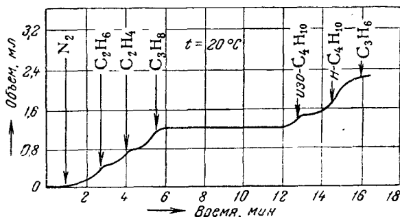
Рис. 2. Интегральная хроматограмма разделения углеводородов методом Янака на цеолите. Температура колонки 20 °C.
