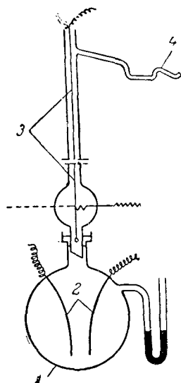
Рис. VIII, 7. Схема прибора для изучения термической диссоциации воды:
