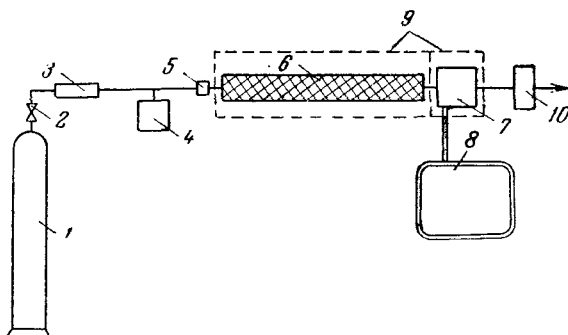
Рис. 1. Схема хроматографа:
