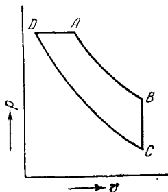
Рис. 1, 6. Цикл Дизеля.
