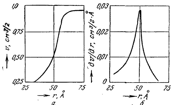
Рис. XIX, 8. Структурная кривая (а) и кривая распределения объема пор по значениям эффективных радиусов (б) для силикагеля.
