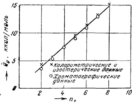
Рис. 15. Зависимость теплот адсорбции Q_a n -алканов на графитированной саже от числа атомов углерода n_c в их молекуле, полученная разными методами.
