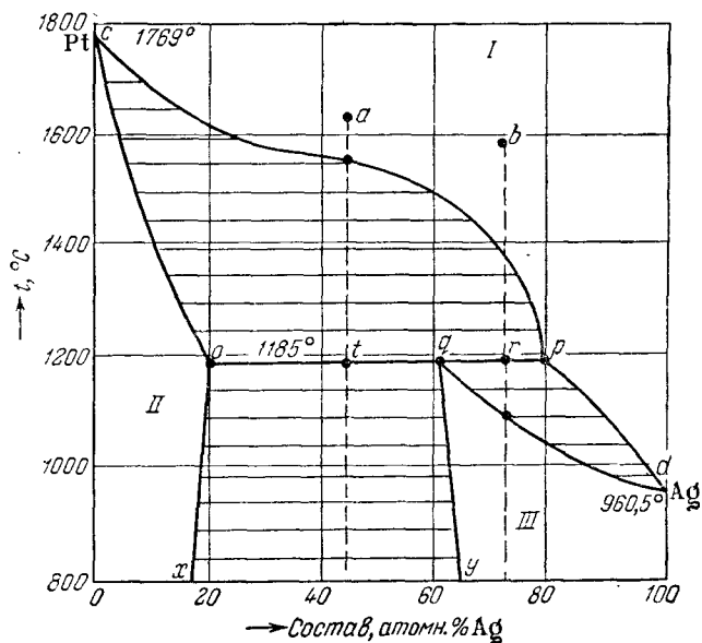
Рис. XIV, 8. Диаграмма плавкости системы платина—серебро.
