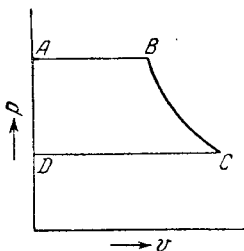
Рис. 1, 5. Цикл Рэнкина.
