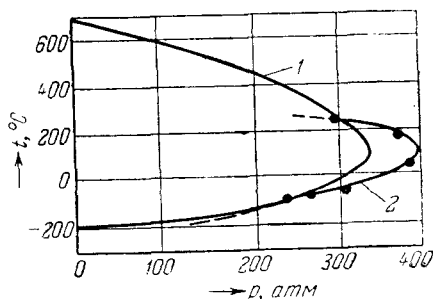
Рис. IV, 13. Инверсионные кривые для воздуха:
