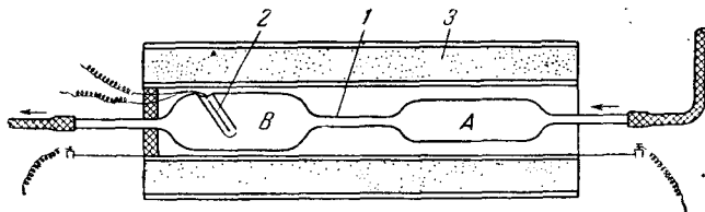
Рис. VIII, 6. Схема реакционного сосуда для изучения гомогенной каталитической реакции:
