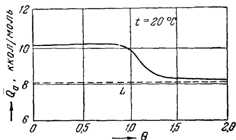
Рис. XVI, 8. Зависимость дифференциальной теплоты адсорбции \bar{Q}_d пара бензола от заполнения поверхности графитированной сажи \theta .
