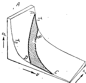
Рис. I, 3. Цикл Карно.
