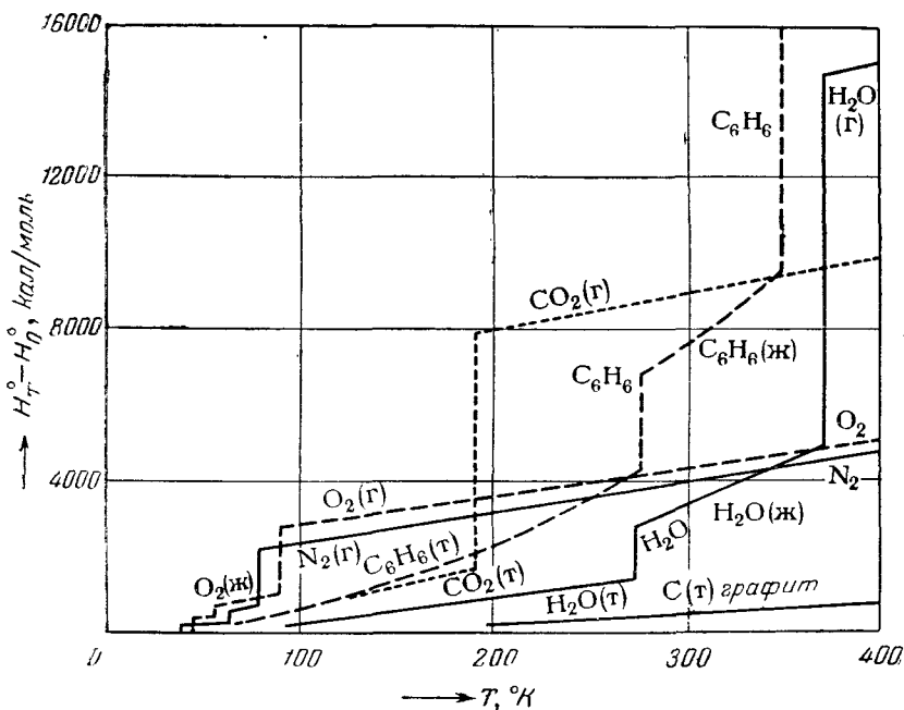
Рис. 1, 7. Прирост энтальпии некоторых веществ как функция температуры.
