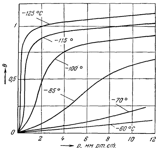
Рис. XVI, 5. Изотермы адсорбции этана на поверхности графитированной сажи при разных температурах.
