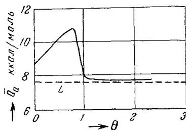
Рис. XVI, 10. Зависимость дифференциальной теплоты адсорбции \bar{Q}_a пара четыреххлористого углерода от заполнения \theta поверхности графитированной сажи.
