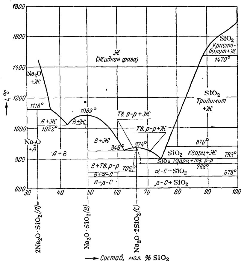
Рис. XIV, 16. Диаграмма состояния силиката окись натрия—диоксид кремния.
