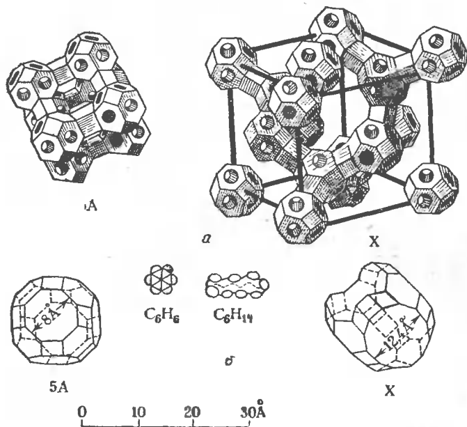
Рис. XIX, 1. Модели решеток (а) и полостей (б) пористых кристаллов цеолитов типа А и Х (фожазит).
