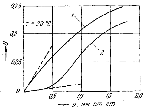
Рис. XVI, 1. Изотермы адсорбции на поверхности графитированной сажи в области невысоких заполнений \theta поверхности и небольших равновесных давлений p в газовой фазе:
