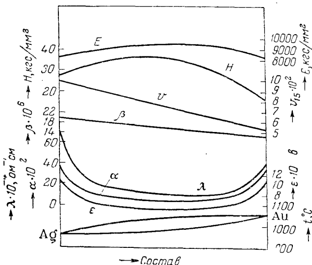
Рис. XIV, 9. Диаграмма зависимости свойств сплава золото—серебро от состава:
