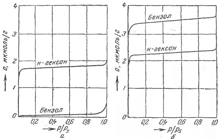
Рис. XIX, 2. Изотермы адсорбции паров бензола и n -гексана пористыми кристаллами цеолитов: а—типа 5А; б—типа 13Х (Na-фожазит).
