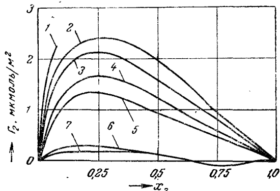
Рис. XIX, 11. Изотермы адсорбции на крупнопористом силикагеле с гидроксильрованной поверхностью из растворов в предельном углеводороде: 1—нафталина; 2—бензола; 3—толуола; 4—циклогексана; 5—гептена-1; 6—циклогексана; 7—метилциклогексана.
