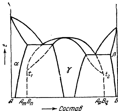
Рис. XIV, 12. Схема, поясняющая образование бертоллидов в случае иррационального максимума на кривой плавления.
