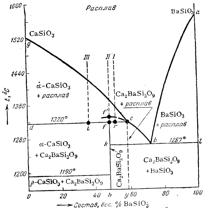
Рис. XIII, 10. Диаграмма состояния двухкомпонентной системы \text{CaSiO}_3 - \text{BaSiO}_3 , образующей химическое состояние, плавящееся инконгруентно.
