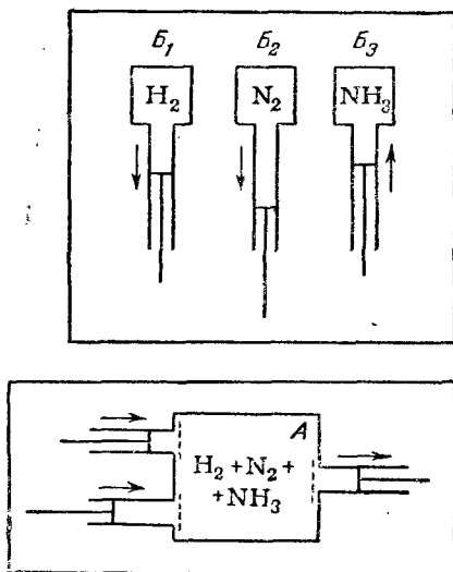
Рис. VIII, 1. Ящик Вант-Гоффа.
