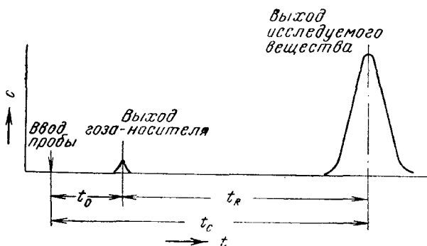
Рис. 8. Схема, иллюстрирующая отсчет времени удерживания:
