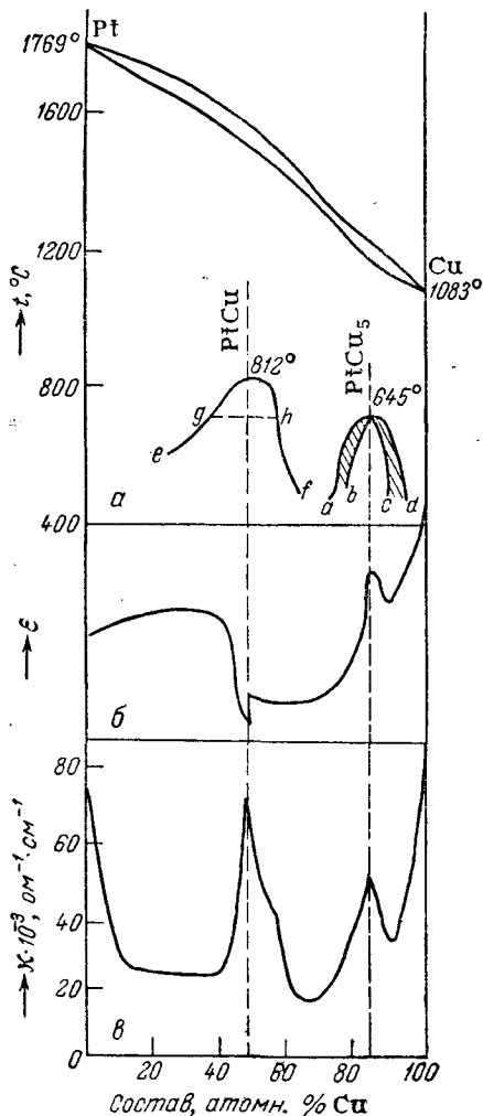
Рис. XIV, 13. Система платина—медь: а —диаграмма плавкости; б —зависимость термоэлектродвижущей силы (в сочетании со свинцом) от состава; в —зависимость удельной электропроводности от состава.
