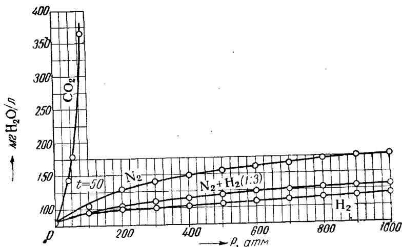
Рис. IV, 11. Зависимость концентрации насыщенного пара \text{H}_2\text{O} в сжатых газах от общего давления.
