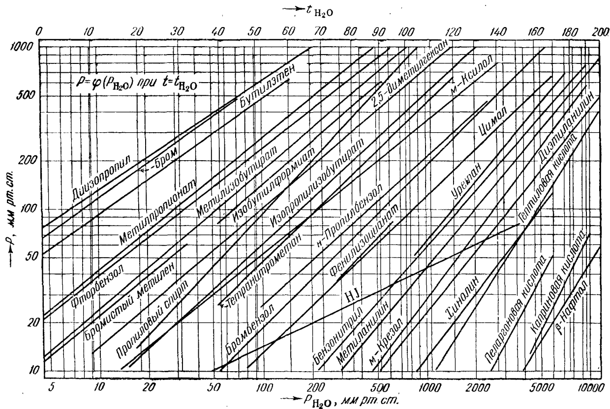
Рис. IV, 9. Давления насыщенного пара некоторых жидкостей как функции давления насыщенного пара воды ( t=t_{H_2O} ).
