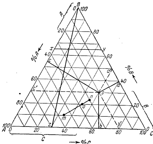
Рис. XV, 1. Треугольник Гиббса—Розебома для выражения состава трехкомпонентной системы.
