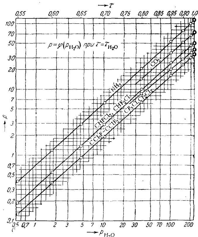
Рис. IV, 10. Давления насыщенного пара некоторых жидкостей как функции давления насыщенного пара воды ( T=T_{H_2O} ).
