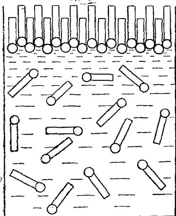
Рис. XVII, 6. Схема «частокола Лэнгмюра» при адсорбции на поверхности водный раствор—пар молекул поверхностноактивного вещества из водного раствора.
