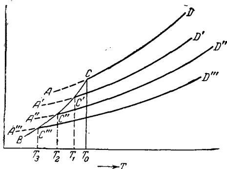
Рис. VII, 3. Понижение температуры затвердевания растворов.
