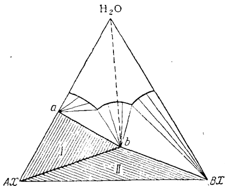
Рис. XV. 9. Треугольная фазовая диаграмма ( T=\text{const} ) системы, состоящей из воды и двух солей с общим ионом.
