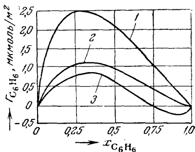
Рис. XIX, 10. Изотермы гиббсовской адсорбции \Gamma_{\text{C}_6\text{H}_6} бензола из растворов с n -гексаном:
