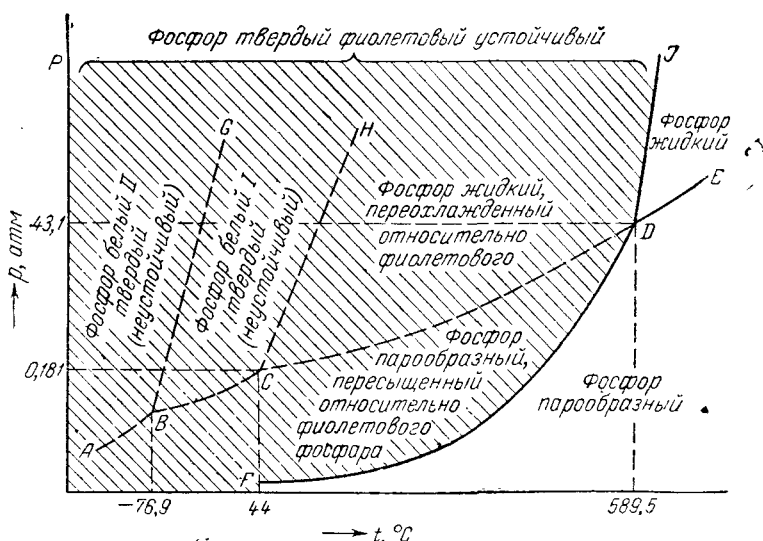
Рис. XII, 7. Диаграмма состояния фосфора.
