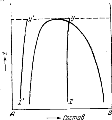
Рис. XIV, 3. Составы жидких фаз и состав паровозной фазы при различных температурах.
