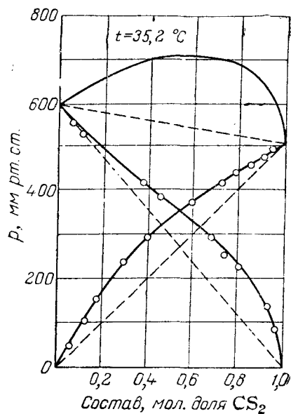
Рис. VI, 11. Давление пара системы сероуглерод—метилаль.
