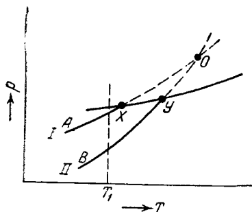
Рис. XII, 6. Диаграмма состояния бензофенона.
