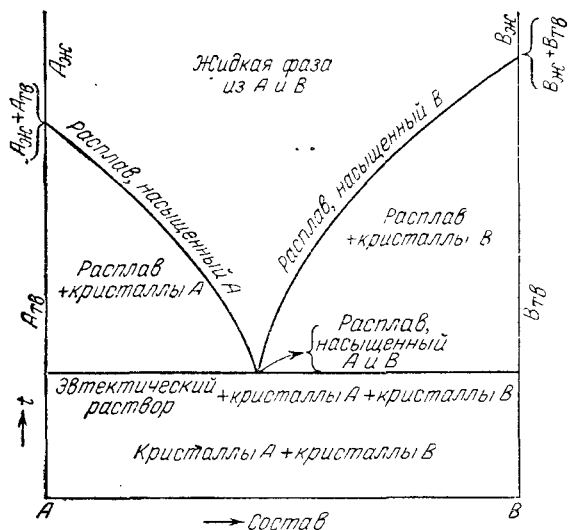
Рис. XIII, 14. Диаграмма, иллюстрирующая принцип соответствия.
