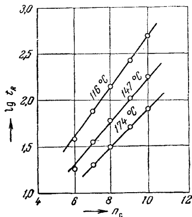
Рис. 11. Зависимость логарифма исправленного времени удерживания различных n -алканов от числа атомов углерода ( n_C ) в их молекуле.
