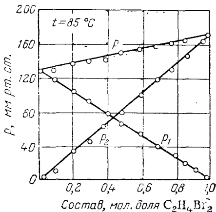
Рис. VI, 2. Давление пара раствора: дибромпропан—дибромэтан.
