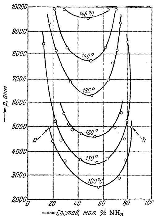
Рис. V, 7. Ограниченная взаимная растворимость газообразных N_2 и NH_3 .
