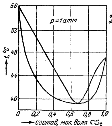
Рис. VI, 13. Диаграмма температуры кипения—состав бинарной смеси с минимумом температуры кипения (метилаль—сероуглерод).
