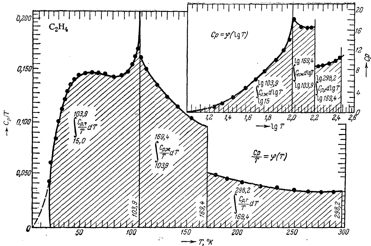
Рис. III. 3. Графическое вычисление энтропии этилена.
