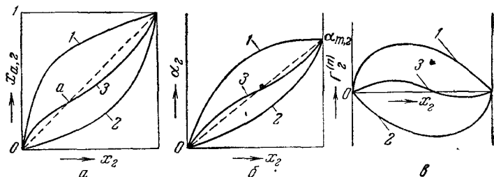
Рис. XIX, 9. Зависимость от состава объемного раствора ( x_2 ): а—состава поверхностного раствора x_{a,2} ; б—поверхностной концентрации \alpha_2 ; в—гиббсовской адсорбции \Gamma_2(n) .
