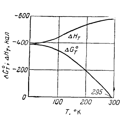
Рис. IX, 3. Зависимость \Delta G_T^\circ и \Delta H_T процесса \text{Sn}(\beta) = \text{Sn}(\alpha) от температуры.
