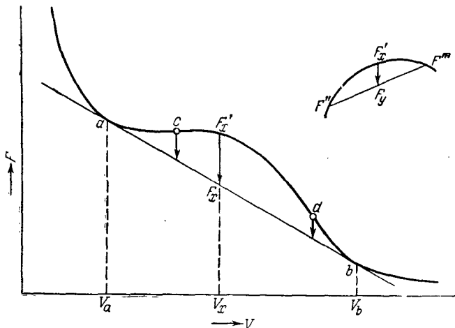
Рис. XII, 8. Изменение изохорного потенциала при переходе вещества из одного агрегатного состояния в другое.
