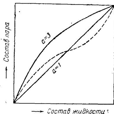
Рис. VI, 3. Составы жидкости и пара бинарного идеального раствора.
