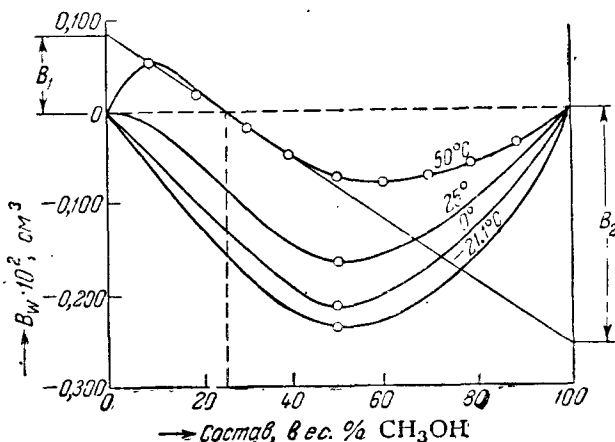
Рис. V, 6. Зависимость объемного эффекта образования раствора C_7H_8-CH_3OH от состава раствора.
