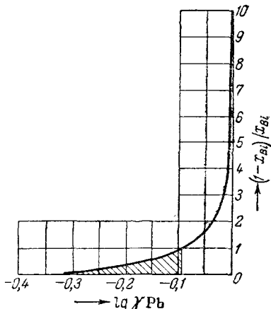
Рис. VI, 20. Графическое вычисление коэффициента активности второго компонента.
