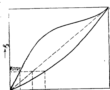
Рис. VII, 1. Парциальное давление газа над его растворами.
