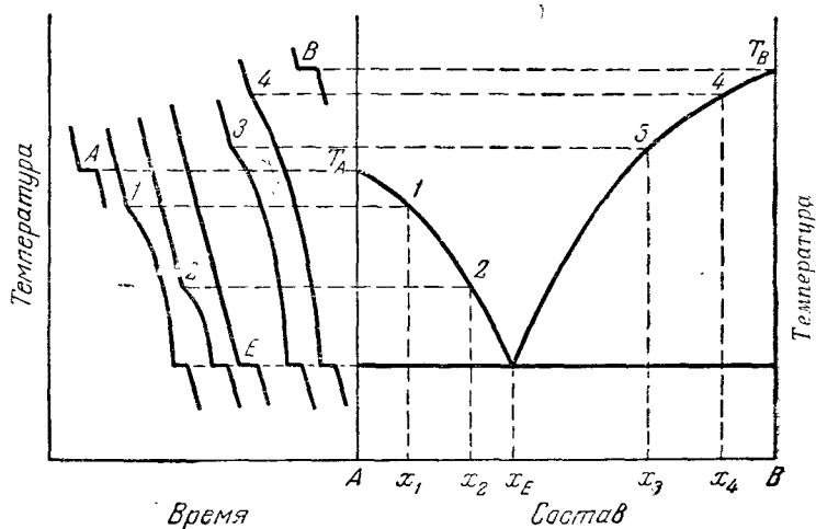
Рис. XIII, 4. Построение диаграммы состояния двухкомпонентной системы по кривым охлаждения.
