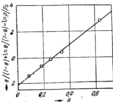
Рис. XVII, 12. Изотерма адсорбции \text{NH}_3 при -78^\circ\text{C} на однородной поверхности графитированной сажи (см. рис. XVII, 11), представленная в координатах линейной формы (XVII, 466) уравнения изотермы мономолекулярной нелокализованной адсорбции Хилла.
