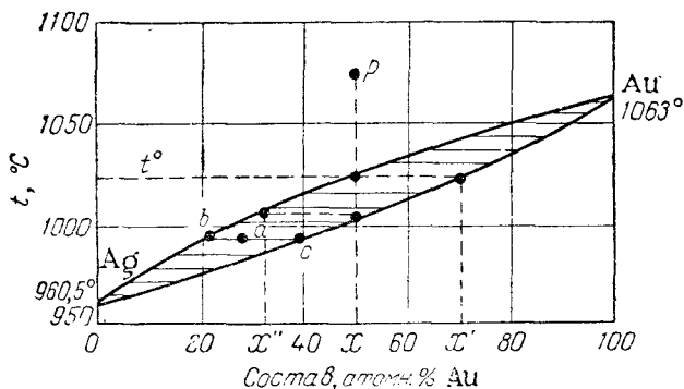
Рис. XIV, 5. Диаграмма плавкости системы золото—серебро.
