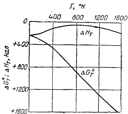
Рис. IX, 4. Зависимость \Delta G_T^\circ и \Delta H_T процесса \text{C}(\text{графит}) = \text{C}(\text{алмаз}) от температуры.
