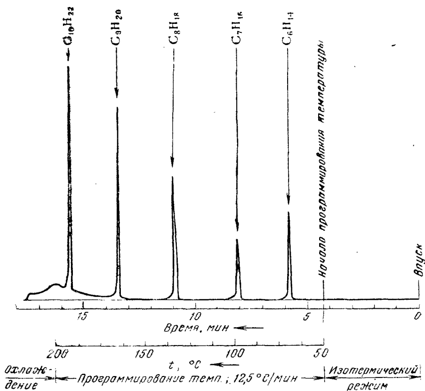
Рис. 12. Разделение углеводородной смеси с применением программированного подъема температуры.
