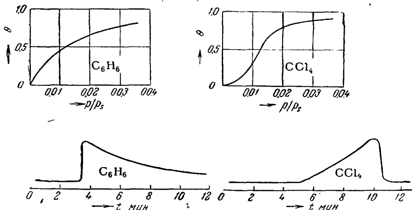
Рис. 7. Изотермы адсорбции C_6H_6 и CCl_4 на однородной поверхности графитированной сажи и соответствующие хроматограммы.
