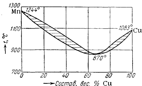
Рис. XIV, 6. Диаграмма плавкости системы марганец—медь.
