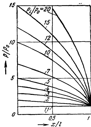
Рис. 14. Изменение давления газа вдоль колонки, при разных значениях p_i/p_o .
