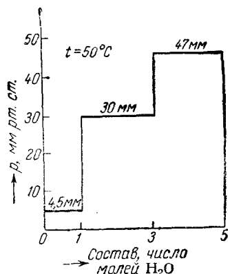
Рис. XIII, 12. Зависимость давления пара воды от состава равновесных с ним кристаллогидратов.
