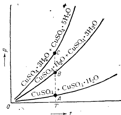
Рис. XIII, 11. Зависимость от температуры давления пара воды, находящегося в равновесии с кристаллогидратами сульфата меди.
