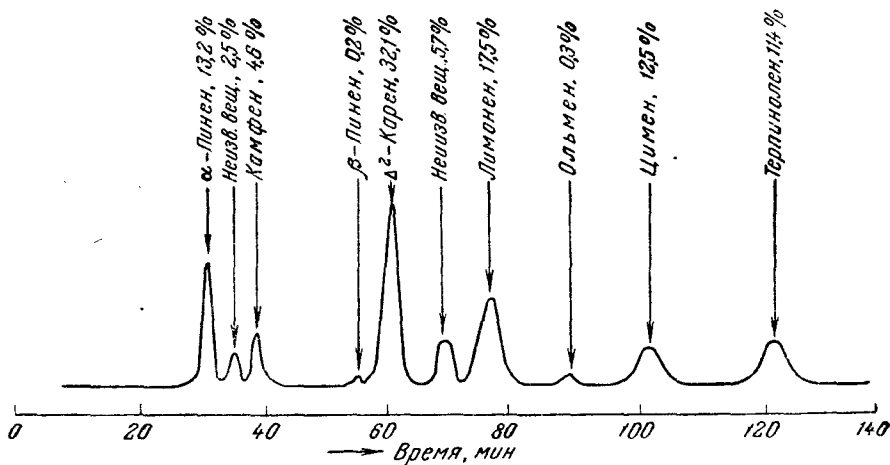
Рис. 3. Дифференциальная хроматограмма смеси терпенов. Неподвижная жидкость—трикрезилфосфат, температура колонки 100 °С.
