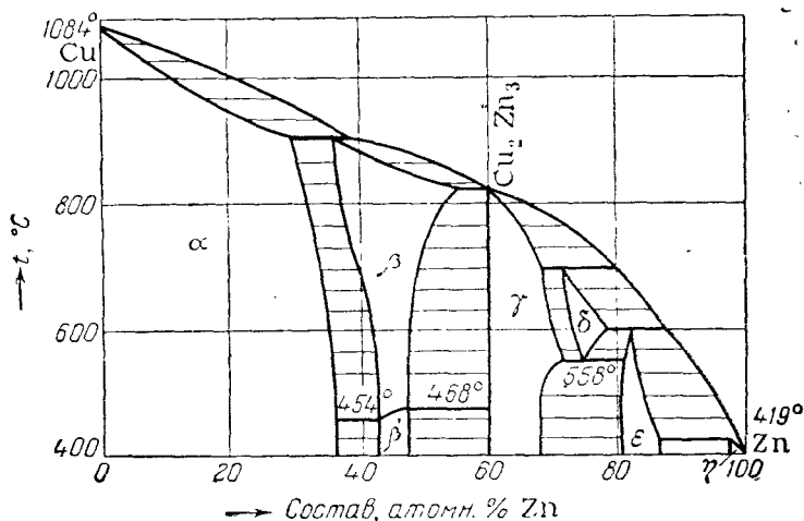
Рис. XIV, 15. Диаграмма состояния системы медь—цинк.
