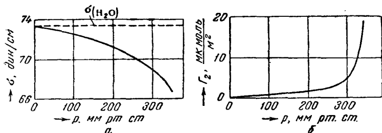
Рис. XVII, 5. Зависимость от парциального давления n -пентана в газовой фазе:
