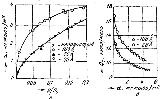
Рис. XIX. 3. Изотермы адсорбции паров бензола гидроксилированными образцами кремнезема с различными размерами пор (а) и соответствующие зависимости дифференциальной теплоты адсорбции от величины адсорбции (б).
