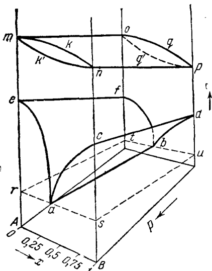
Рис. XIII, 1. Объемная диаграмма состояния двухкомпонентной системы с одной эвтектикой и без твердых растворов.
