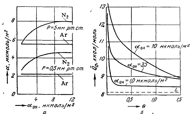
Рис. XVIII, 7. Зависимость величины адсорбции \alpha азота и аргона от концентрации \alpha_{OH} гидроксильных групп на поверхности кремнезема при различных равновесных давлениях в газовой фазе (а) и дифференциальных теплот адсорбции \bar{Q}_d пара бензола от заполнения \theta поверхностей кремнезема, содержащих различные количества гидроксильных групп (б).
