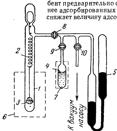
Рис. XVI, 12. Схема определения величины адсорбции с помощью весов Мак-Бэна—Багра:
