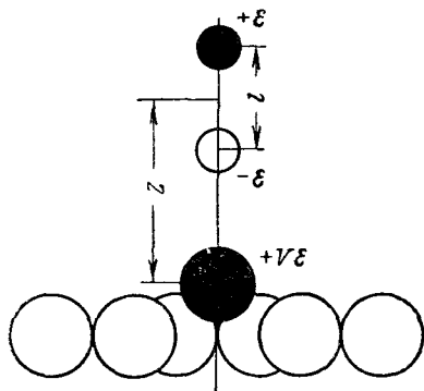
Рис. XVIII, 5. Схема взаимодействия молекулы адсорбата, обладающей диполем \mu_2 = \varepsilon l , с «изолированным» катионом v\varepsilon поверхности.
