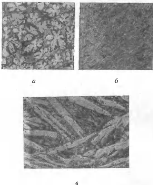
Рис. XIII, 3. Микрофотографии сплавов камфоры с м -нитроанилином:
