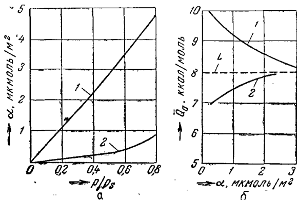
Рис. XVIII, 9. Изотермы адсорбции пара \text{CCl}_4 (а) и зависимость дифференциальной теплоты адсорбции этого пара от величины адсорбции (б) на кремнеземе: 1—на гидроксильной поверхности; 2—на триметилсилированной поверхности. L—теплота конденсации.
