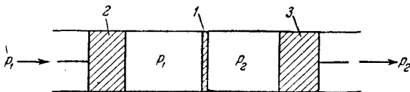
Рис. IV, 12. Схема опыта Джоуля—Томсона.
