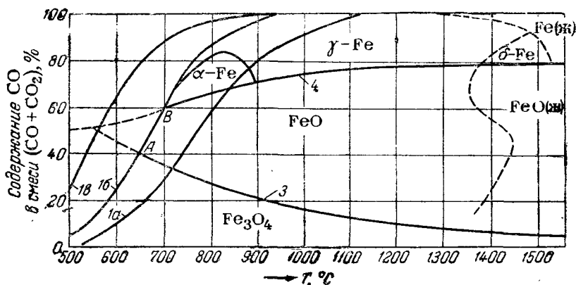
Рис. IX. 1. Равновесие окислов углерода с окислами железа.
