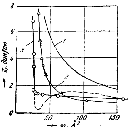
Рис. XVII, 13. Кривые уравнения состояния адсорбированных слоев на поверхности графитированной сажи при -78^\circ\text{C} : 1 — идеальный двумерный газ; 2 — \text{SF}_6 ; 3 — \text{NH}_3 .
