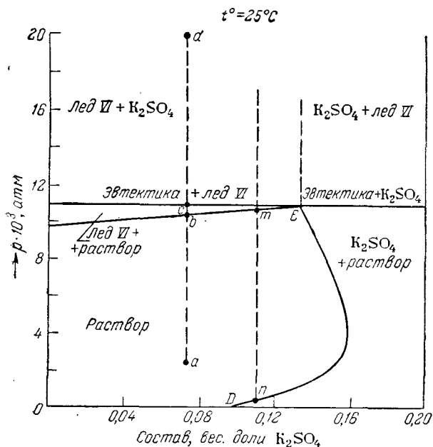
Рис. XIII, 6. Диаграмма состояния двухкомпонентной системы H_2O-K_2SO_4 в осях давление—процентный состав.
