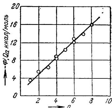
Рис. XVIII, 3. Зависимость (вычисленная) потенциальной энергии адсорбции n -алканов на базисной грани графита от числа n атомов углерода в их молекуле.
