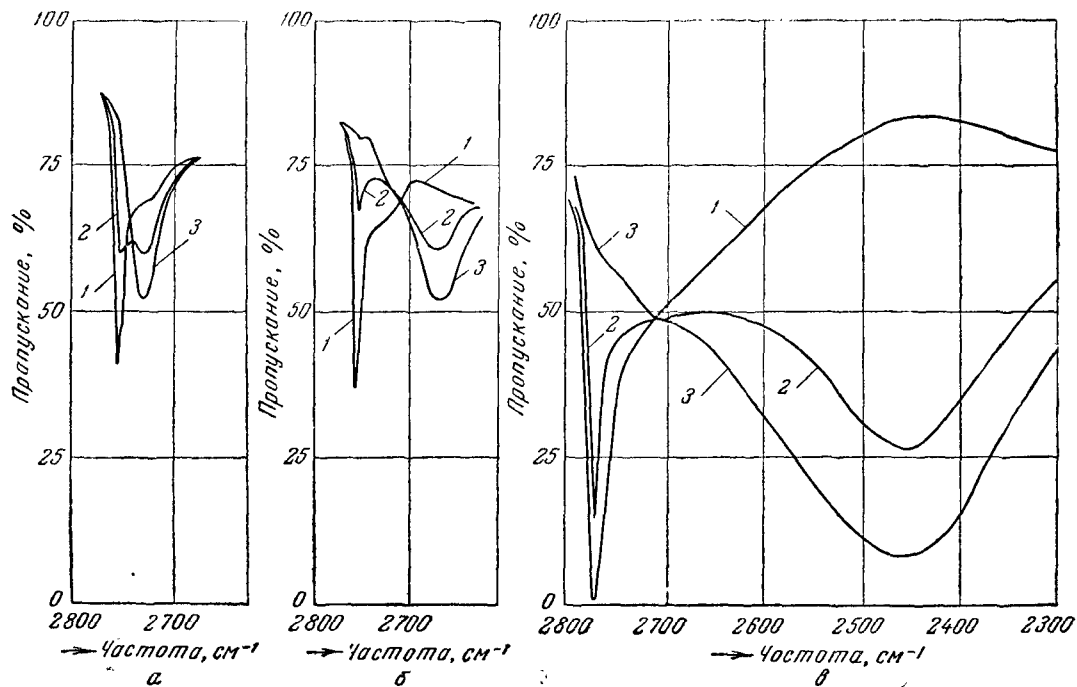
Рис. XVIII, 11. Влияние адсорбции n -гексана (а), бензола (б) и диэтилового эфира (в) на полосу валентных колебаний свободных гидроксильных групп ОД поверхности кремнезема: 1—полоса до адсорбции; 2—полоса после адсорбции малых количеств пара; 3—полоса после адсорбции больших количеств пара.
