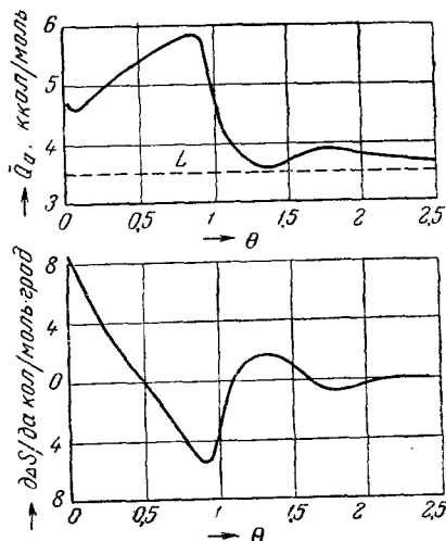
Рис. XVII, 17. Зависимость от заполнения \theta поверхности графитированной сажи дифференциальных теплоты \bar{Q}_a и энтропии \partial \Delta S / \partial a адсорбции этана.
