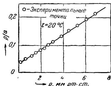
Рис. XVI, 4. Изотерма адсорбции бензола на поверхности графитированной сажи (см. рис. XVI, 1) в координатах линейной формы уравнения Лэнгмюра.
