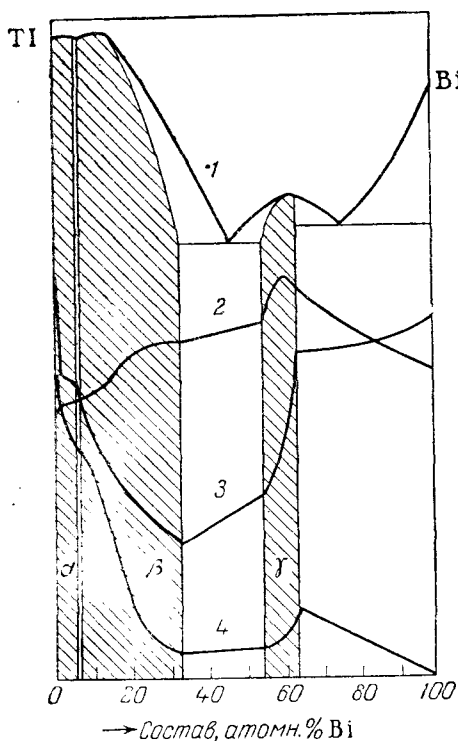
Рис. XIV, 11. Диаграмма состояния системы таллий—висмут:
