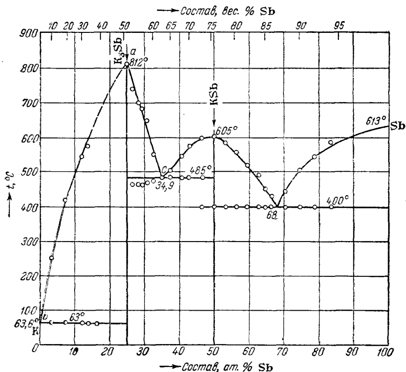
Рис. XIII, 8. Диаграмма состояния двухкомпонентной системы калий—сурьма.
