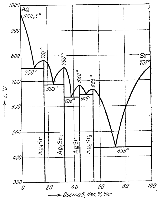
Рис. XIII, 9. Диаграмма состояния двухкомпонентной системы серебро—стронций.
