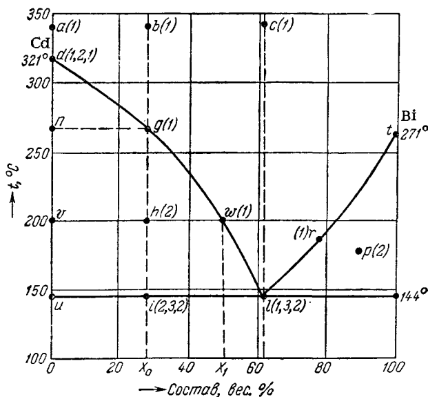
Рис. XIII, 2. Диаграмма состояния двухкомпонентной системы кадмий—висмут.
