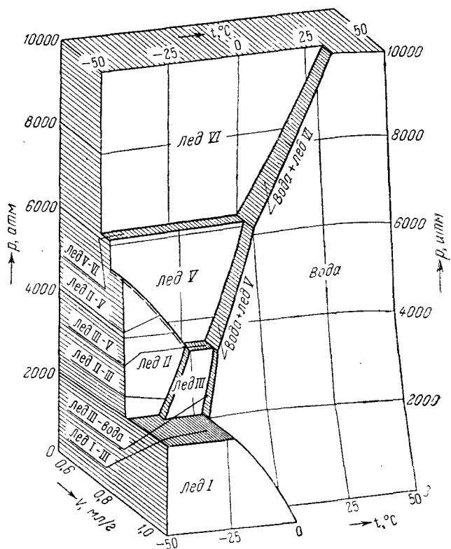
Рис. XII, 3. Объемная диаграмма состояния воды.
