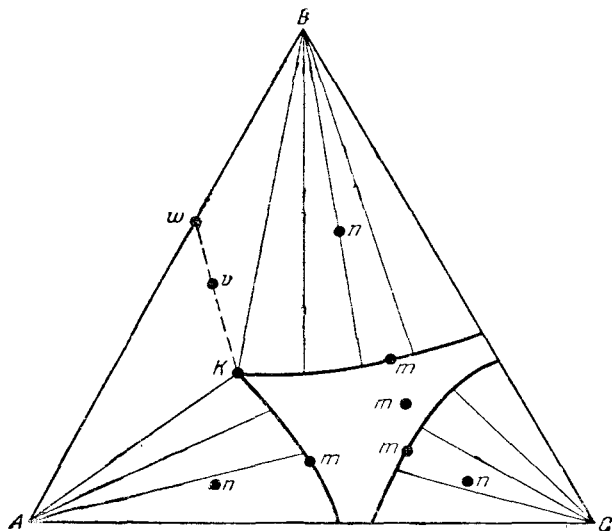
Рис. XV, 4. Сечение объемной треугольной диаграммы плоскостью, отвечающей температуре T_b .
