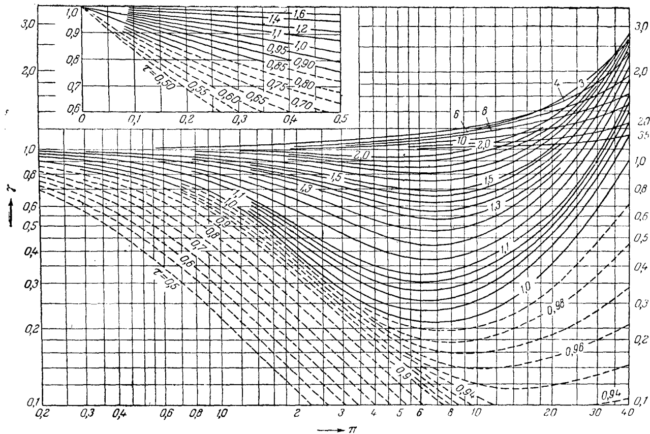
Рис. IV, 4. Зависимость коэффициента активности газов от приведенных давления и температуры.
