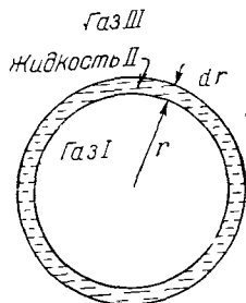
Рис. XVII, 3. Пузырек газа I, отделенный жидкой пленкой II от наружного газа III.
