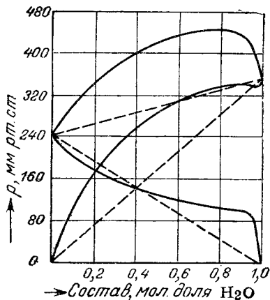
Рис. VI, 6. Давление пара системы \text{C}_5\text{H}_5\text{N}-\text{H}_2\text{O} .
