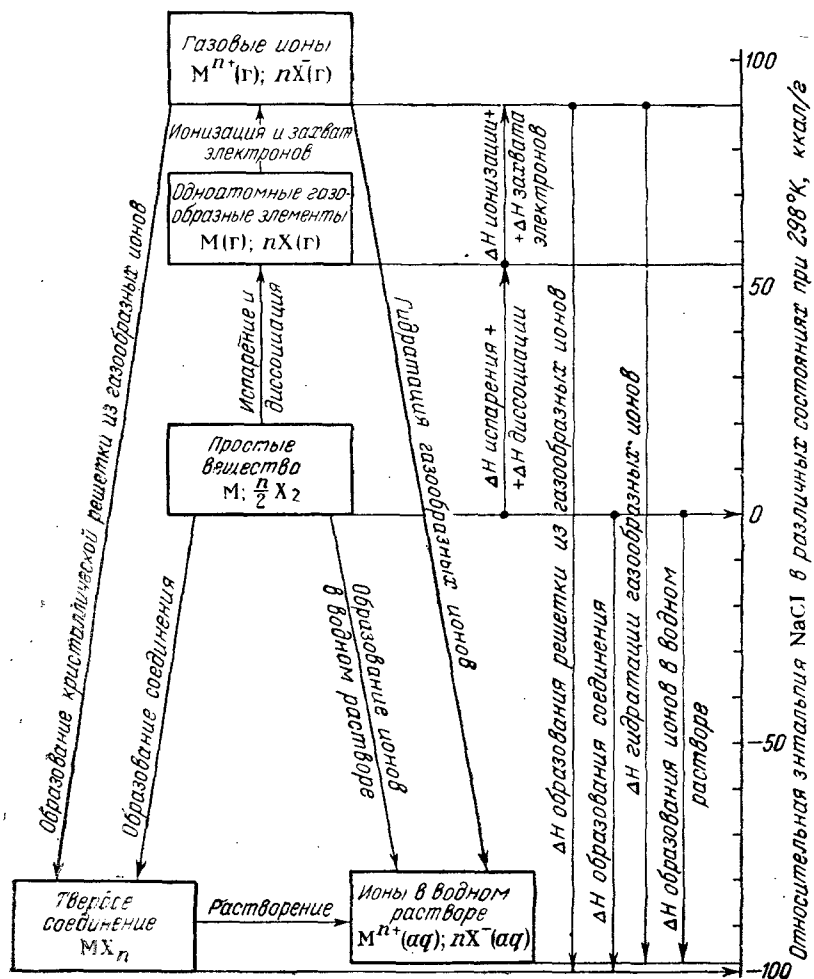
Рис. 11, 2. Термохимические циклы для расчета теплот образования.
