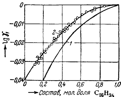
Рис. VII, 9. Зависимость коэффициента активности C_7H_{16} от состава раствора C_7H_{16} — C_{16}H_{34} :
