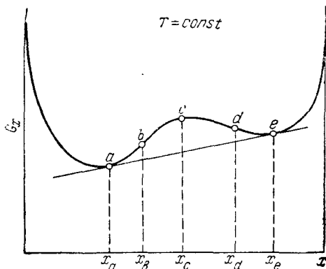
Рис. XII, 9. Изобарный потенциал расслаивающегося раствора.
