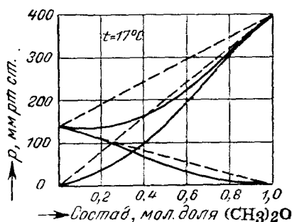
Рис. VI, 5. Давление пара системы (C_2H_5)_2O—CHCl_3 .
