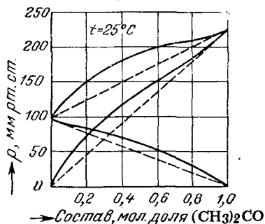
Рис. VI, 4. Давление пара системы C_6H_6-(CH_3)_2CO .
