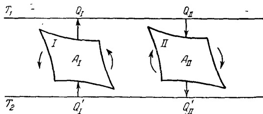
Рис. III, 1. Схема для доказательства теоремы Карно.
