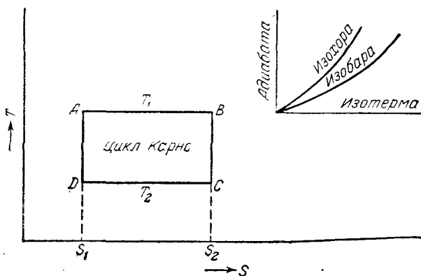
Рис. III, 4. Схема энтропийной диаграммы.
