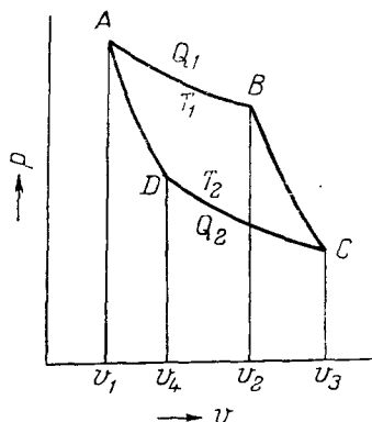
Рис. I, 4. Цикл Карно (проекция на координатную плоскость p-v ).
