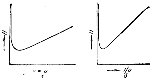
Рис. 19. Графики уравнения ван Димтера а — H=f(u) ; б — H=f(1/u) .
