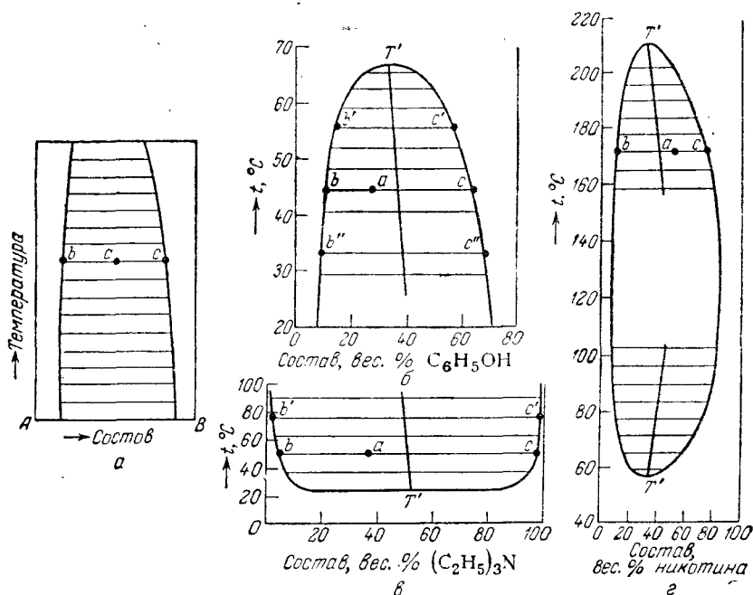
Рис. XIV, 1. Диаграммы состояния расслаивающихся жидких бинарных систем:
