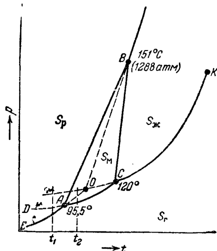
Рис. XII, 5. Диаграмма состояния серы.
