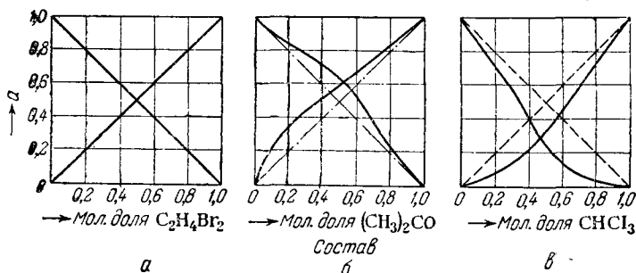
Рис. VI, 18. Активности компонентов бинарных растворов: а— C_2H_6Br_2 - C_2H_4Br_2 (идеальный раствор); б— C_6H_6 - (CH_3)_2CO (положительные отклонения); в— (C_2H_5)_2O - CHCl_3 (отрицательные отклонения).
