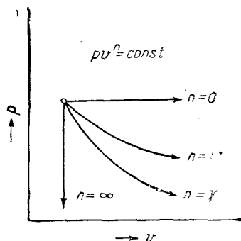
Рис. 1, 8. Простейшие политропные процессы.
