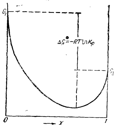
Рис. VIII, 2. Зависимость величины G от химической переменной \chi .
