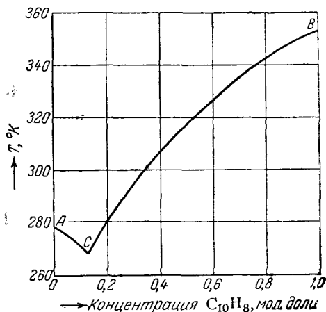
Рис. VII, 4. Температуры затвердевания растворов нафталина в бензоле.
