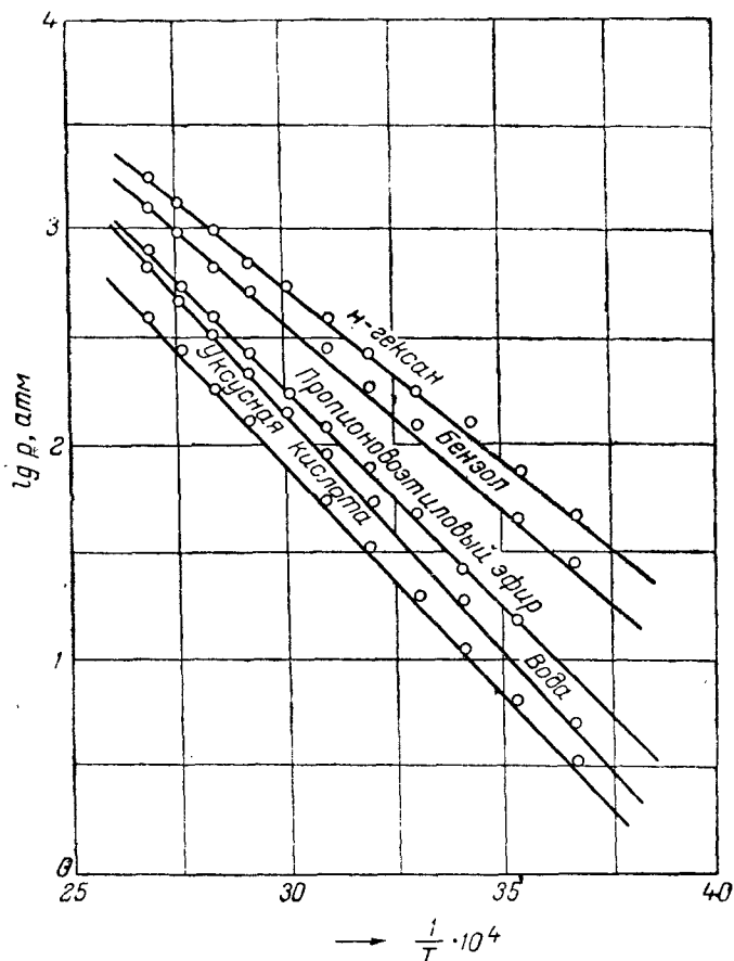
Рис. IV, 8. Зависимость логарифма давления насыщенного пара некоторых жидкостей от обратной температуры.
