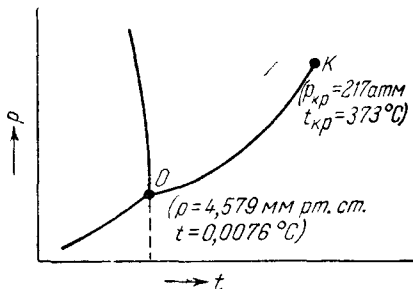
Рис. XII, 4. Плоская диаграмма состояния воды.
