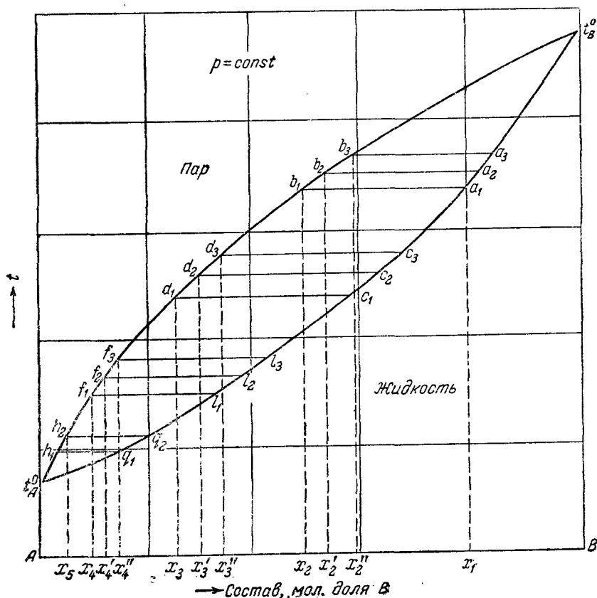
Рис. VI, 9. Диаграмма температура кипения—состав бинарной системы.
