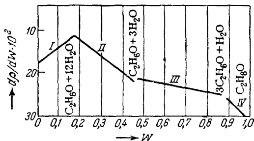
Рис. V, 2. Зависимость производных плотности раствора \text{C}_2\text{H}_5\text{OH}-\text{H}_2\text{O} по составу от весовой доли спирта (по Д. И. Менделееву).
