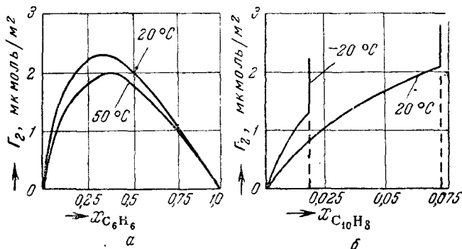
Рис. XIX, 14. Влияние температуры на адсорбцию из бинарных растворов:
