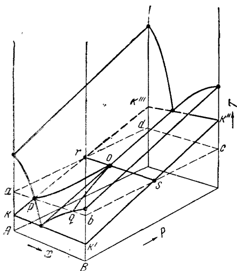
Рис. XIII, 5. Сечение объемной диаграммы двухкомпонентной системы (см. рис. XIII, 1) плоскостью, соответствующей постоянной температуре.
