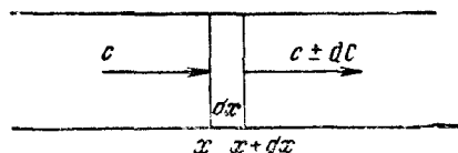
Рис. 5. Изменение концентрации c компонента газовой фазы в поперечном слое газо-хроматографической колонки.
