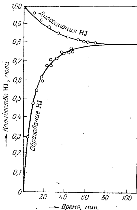
Рис. VIII, 3. Изменение во времени количества \text{HJ} при его образовании и диссоциации.
