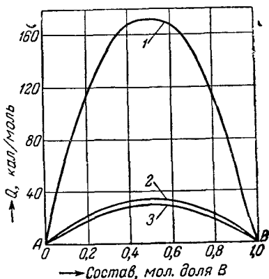
Рис. VII, 7. Зависимость теплоты образования одного моля регулярных растворов от состава:
