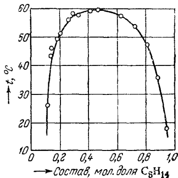
Рис. VI, 17. Ограниченная растворимость в системе \text{C}_6\text{H}_5\text{NH}_2\text{—C}_6\text{H}_{14} .
