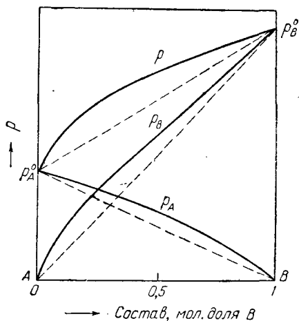
Рис. VI, 1. Полное и парциальные давления пара бинарного раствора.
