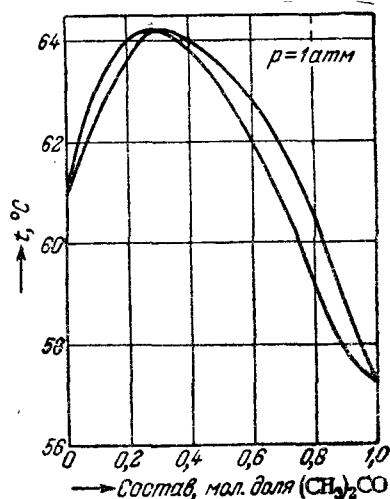
Рис. VI, 14. Диаграмма температуры кипения—состав бинарной смеси с максимумом температуры кипения (хлороформ—ацетон).
