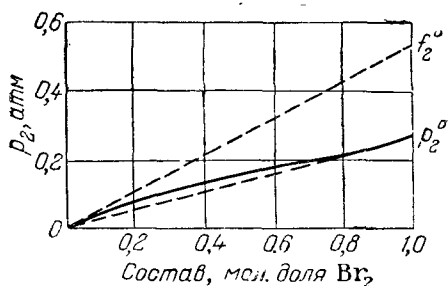
Рис. VI, 19. Давление пара \text{Br}_2 над растворами \text{CCl}_4 - \text{Br}_2 .
