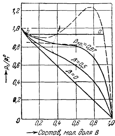
Рис. VI, 16. Зависимость относительного парциального давления компонента от состава раствора.
