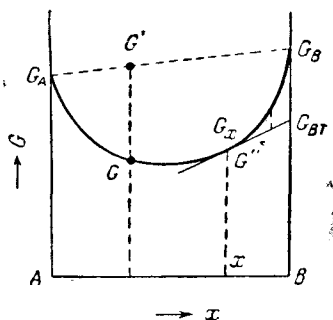
Рис. V, 5. Изобарный потенциал бинарного раствора.
