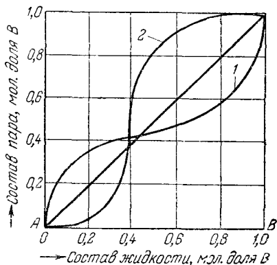
Рис. VI, 15. Изобары x-y : 1—раствор \text{C}_6\text{H}_6-\text{C}_2\text{H}_5\text{OH} ; 2—раствор \text{H}_2\text{O}-\text{HNO}_3 .
