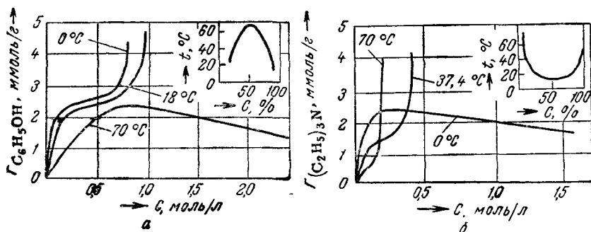
Рис. XIX, 16. Влияние температуры на адсорбцию из расслаивающихся водных растворов:
