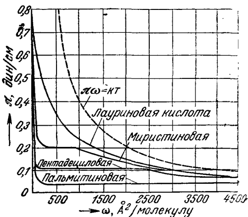
Рис. XVII, 10. Зависимость поверхностного давления \pi монослоев органических кислот от величины площади \omega .
