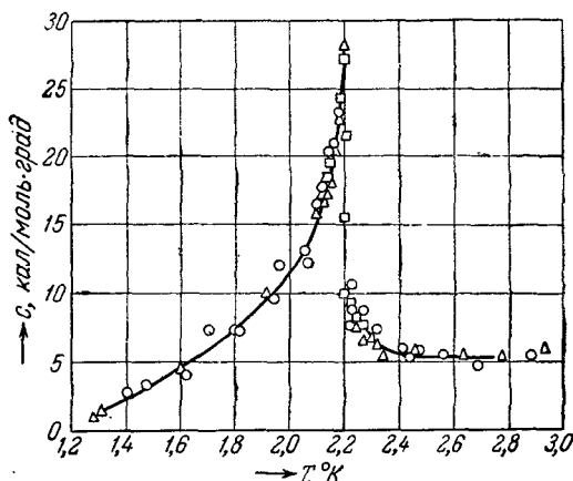
Рис. IV, 5. Зависимость теплоемкости жидкого He от температуры (Кезом и Клузиус).
