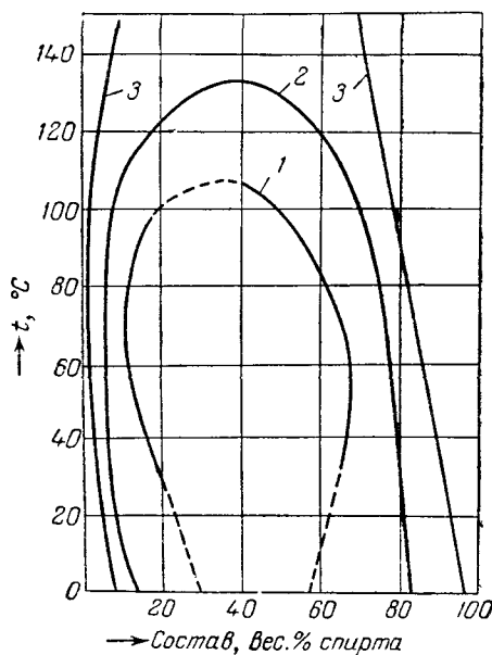
Рис. XIV, 2. Ограниченная взаимная растворимость воды и спиртов:
