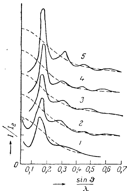
Рис. V. 1. Интенсивность рассеяния рентгеновских лучей жидким аргонном при разных температурах и давлениях:
