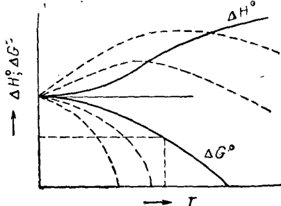
Рис. IX, 2. Зависимости \Delta H^\circ и \Delta G^\circ от температуры.
