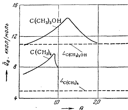
Рис. XVIII, 8. Зависимость дифференциальных теплот адсорбции неопентана и триметилкарбинола от заполнения поверхности графитированной сажи.
