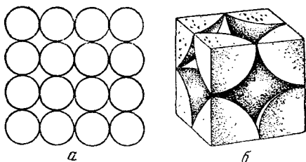
Рис. XIX, 6. Схема поры в адсорбенте глобулярной структуры с координационным числом шесть:
