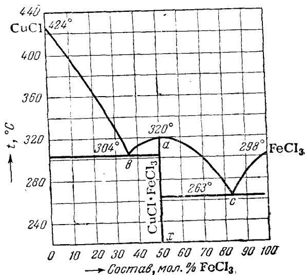
Рис. XIII, 7. Диаграмма состояния двухкомпонентной системы хлористая медь—хлорное железо.
